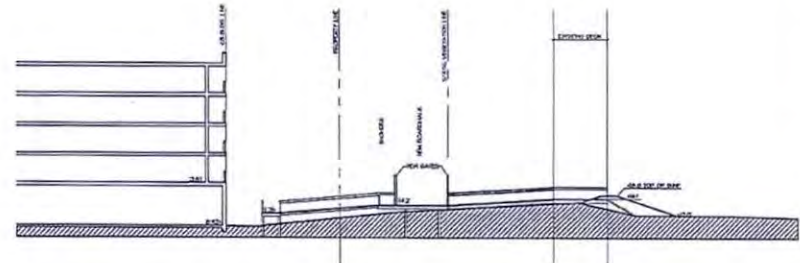
CABANA DEL MAR LONGITUDINAL SECTION SCALE: 1/8" = 1'-0"
