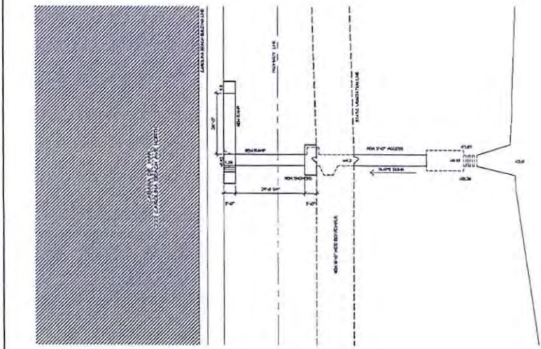
4 CABANA DEL MAR PRELIMINARY SITE LAYOUT SCALE: 1/8" = 1'-0"
